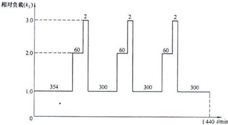
图2 变压器典型负荷曲线
