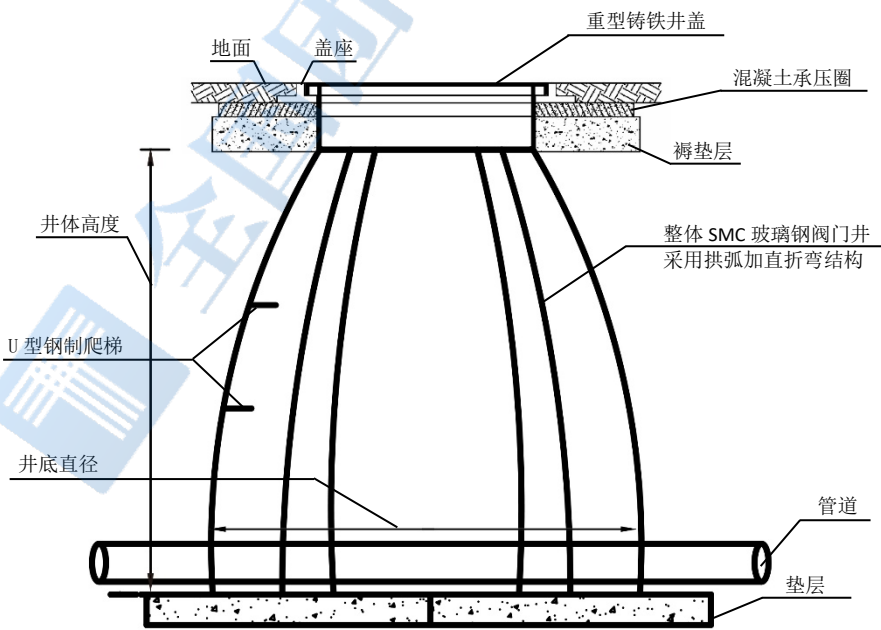
图A.2 B 125 以上安装示意图二
