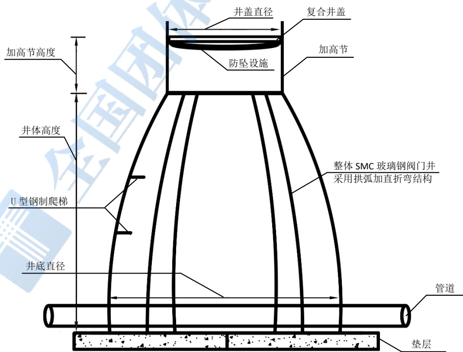
图A.8 B 125 以下安装示意图四
