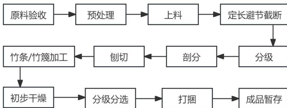
图 1 工艺流程图
