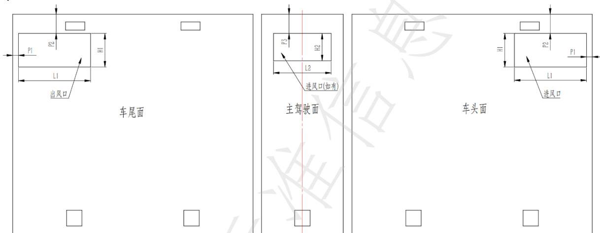
图5 通风口位置示意图
