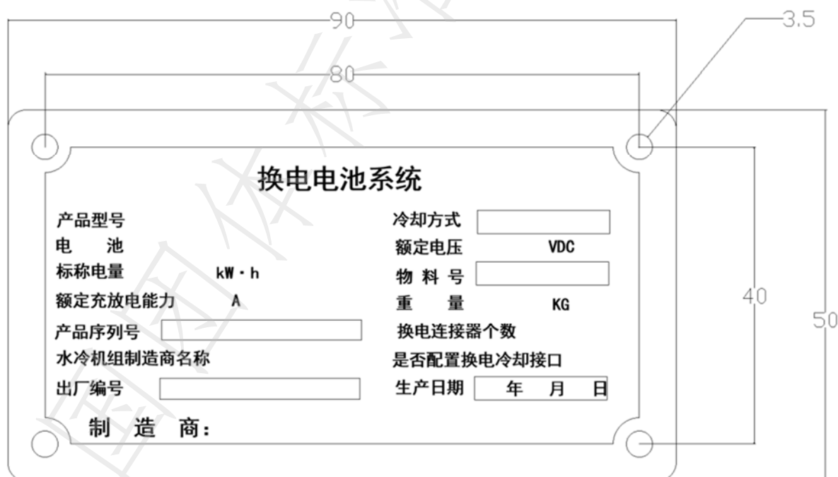
图16 铭牌示例图
