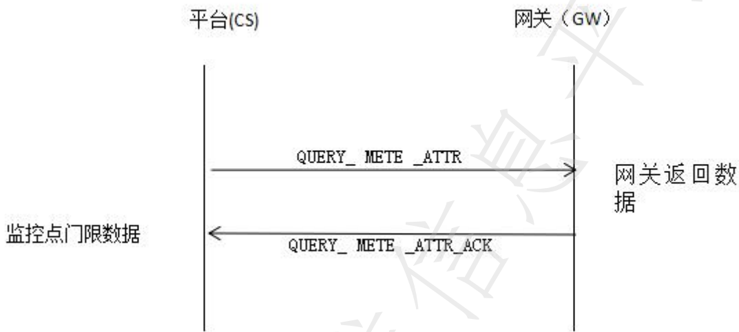
图 A. 6 请求监控量属性
