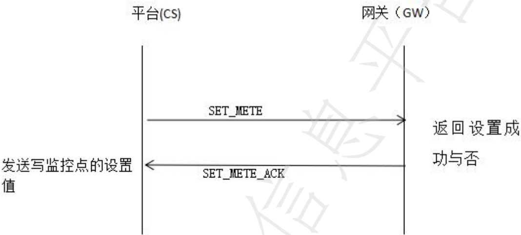
图 A. 5 写监控量设置值（控制）
