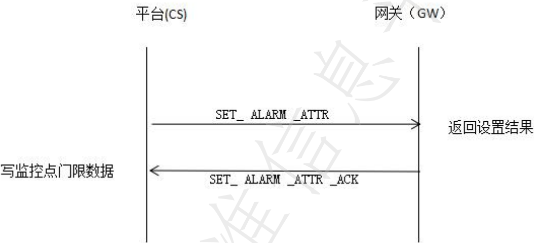
图 A.8 写告警量属性值
