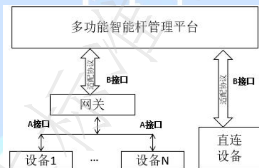
图 2 设备接入示意图
