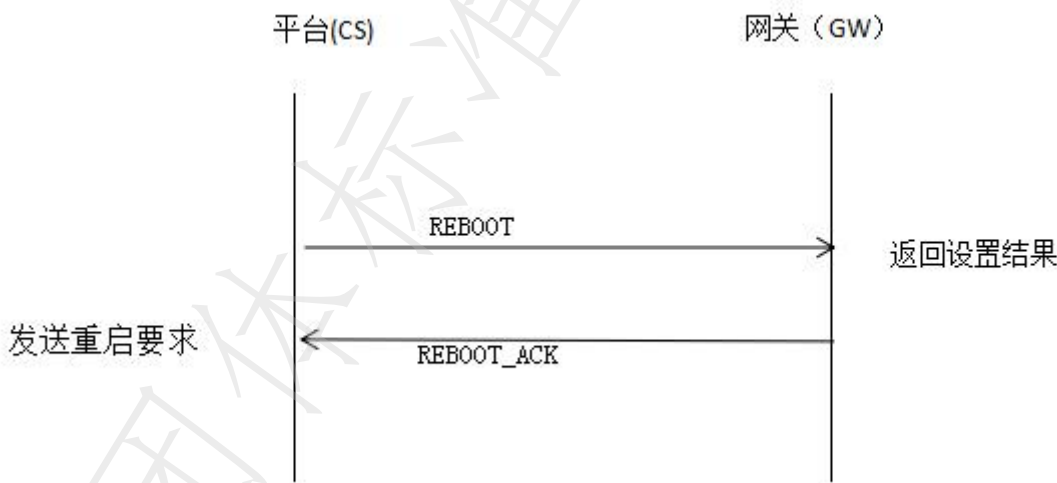
图 A. 10 重启网关 (GW)
