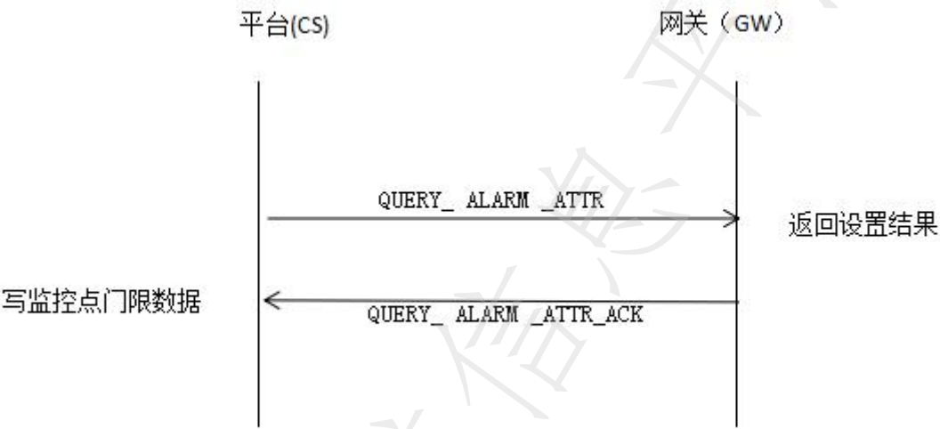
图 A. 9 请求告警量属性值
