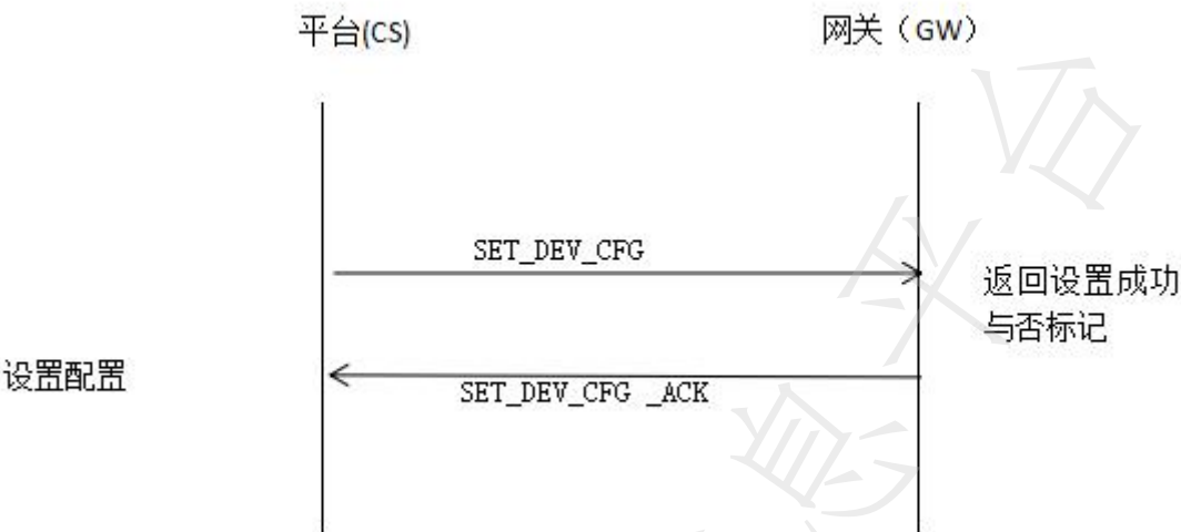
图 A. 13 写配置数据
