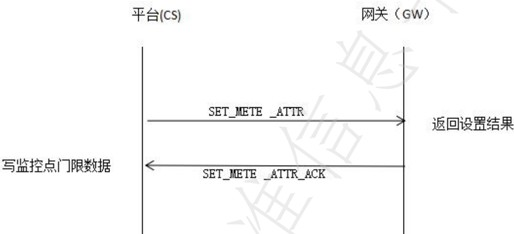
图 A. 7 写监控量属性值
