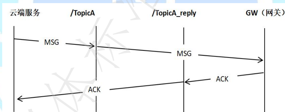
图5 平台向网关下发消息的流程
