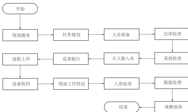
图 A.1 水质监测无人船巡查作业流程
