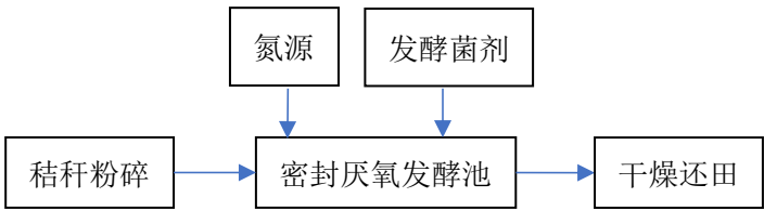
图 2 秸秆厌氧发酵工艺流程
