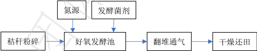
图1 秸秆好氧发酵工艺流程
