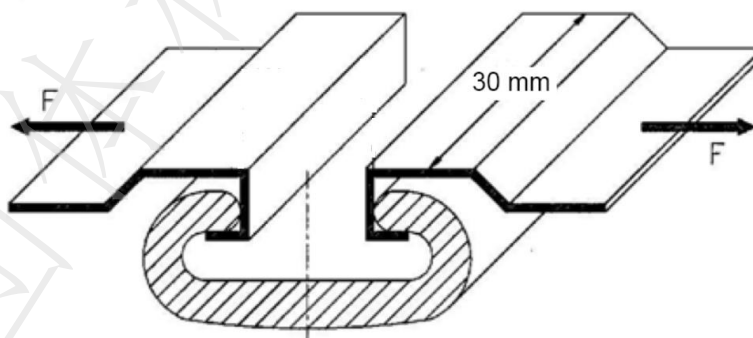
图四 扶手带唇口强度试验
