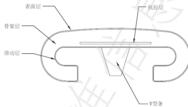
图三 V型扶手带
