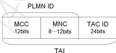
图 8.1.4 跟踪区标识 TAI 编号构成
