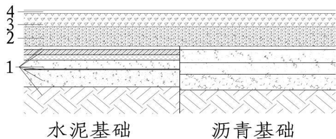
图 1 全单组份湿固化聚氨酯弹性跑道系统构造图
