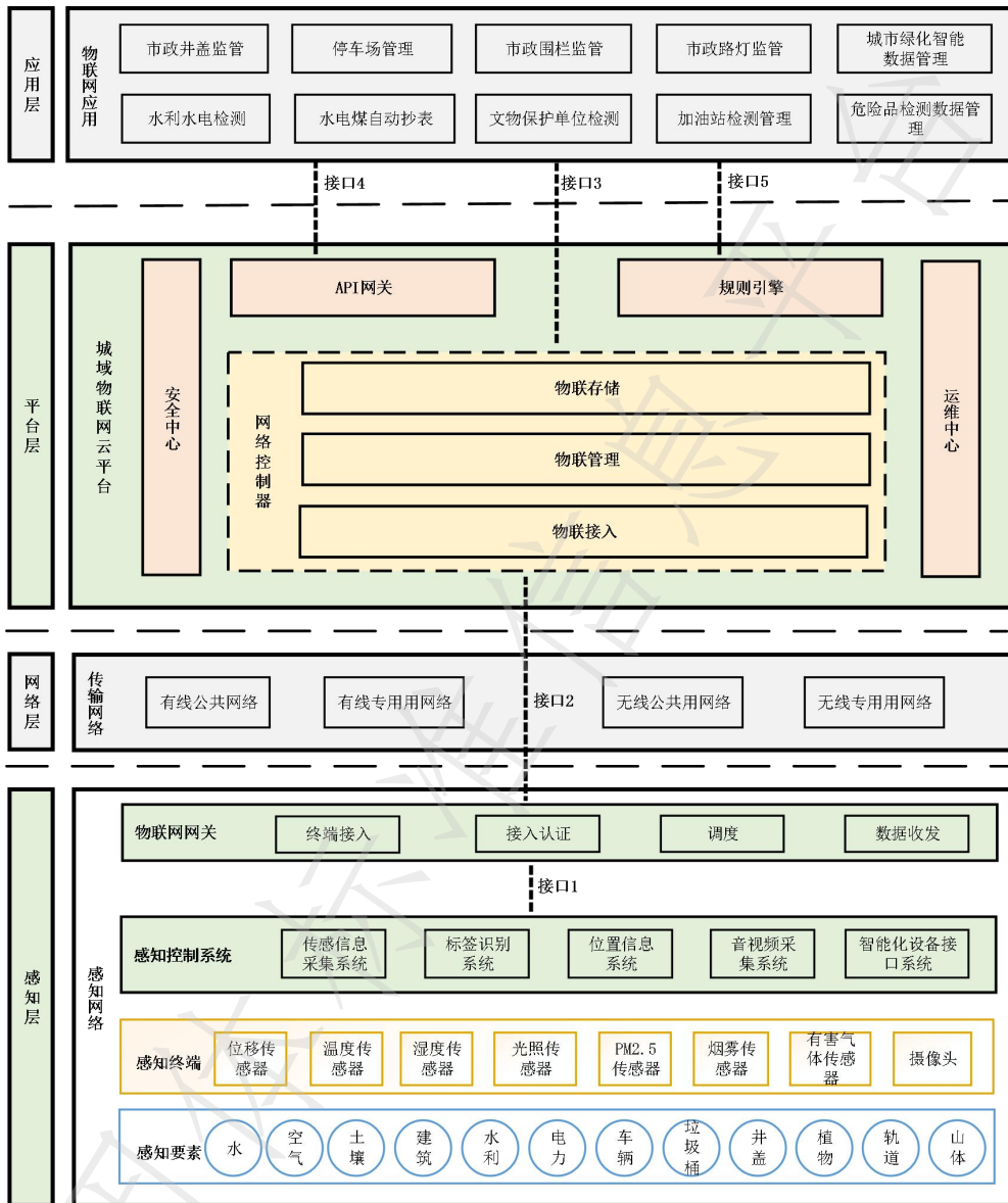
图 1 城域物联感知平台总体参考架构
