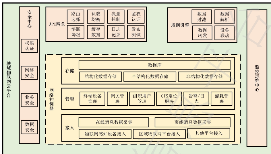
图 2 云平台软件功能参考架构
