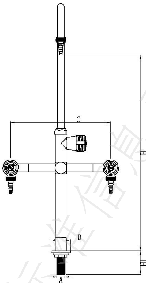
图 A.7 台式三柄三口水龙头
