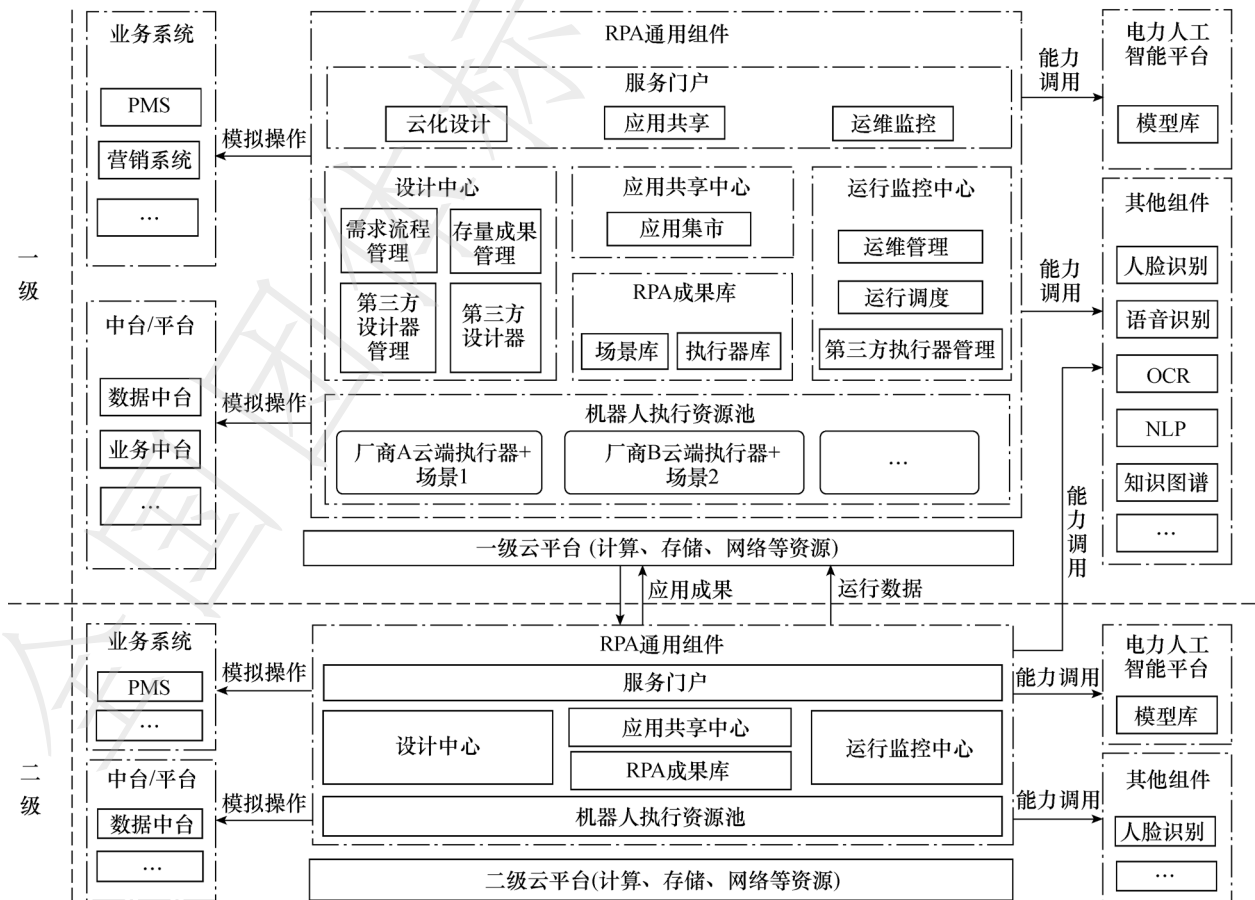
图 1 总体架构图
