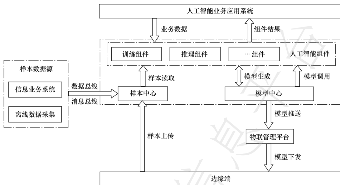
图3 电力人工智能平台数据架构
