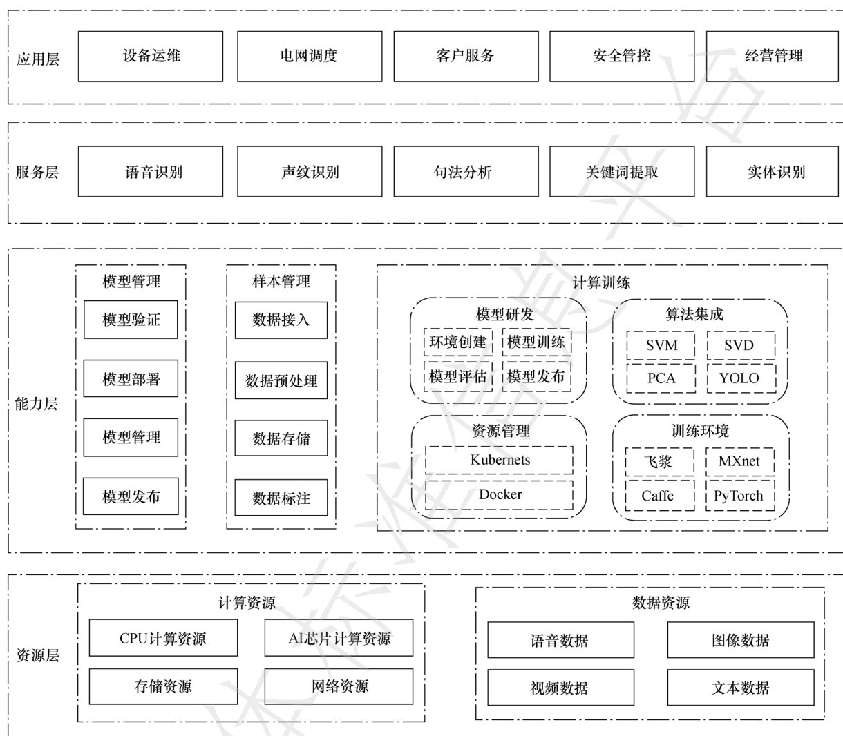
图2 电力人工智能平台技术架构
