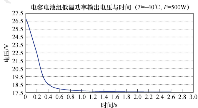
图 B.2 在 -40℃±3℃下 500W 恒功率输出曲线
