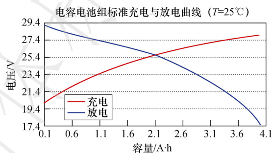
图 B.1 在 25℃±3℃下标准充电与放电曲线
