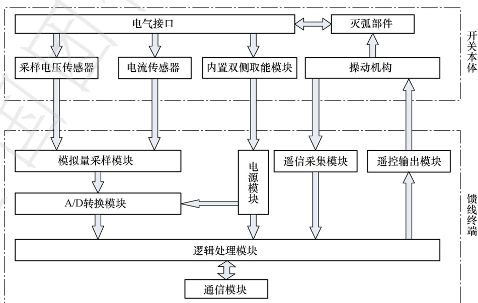
图 A.2 整体设计的 12kV 智能配电柱上开关框图（内部连接）
