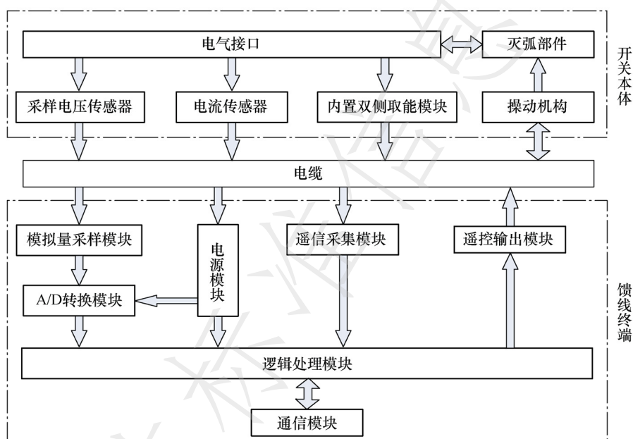
图 A.1 整体设计的 12kV 智能配电柱上开关框图（电缆连接）
