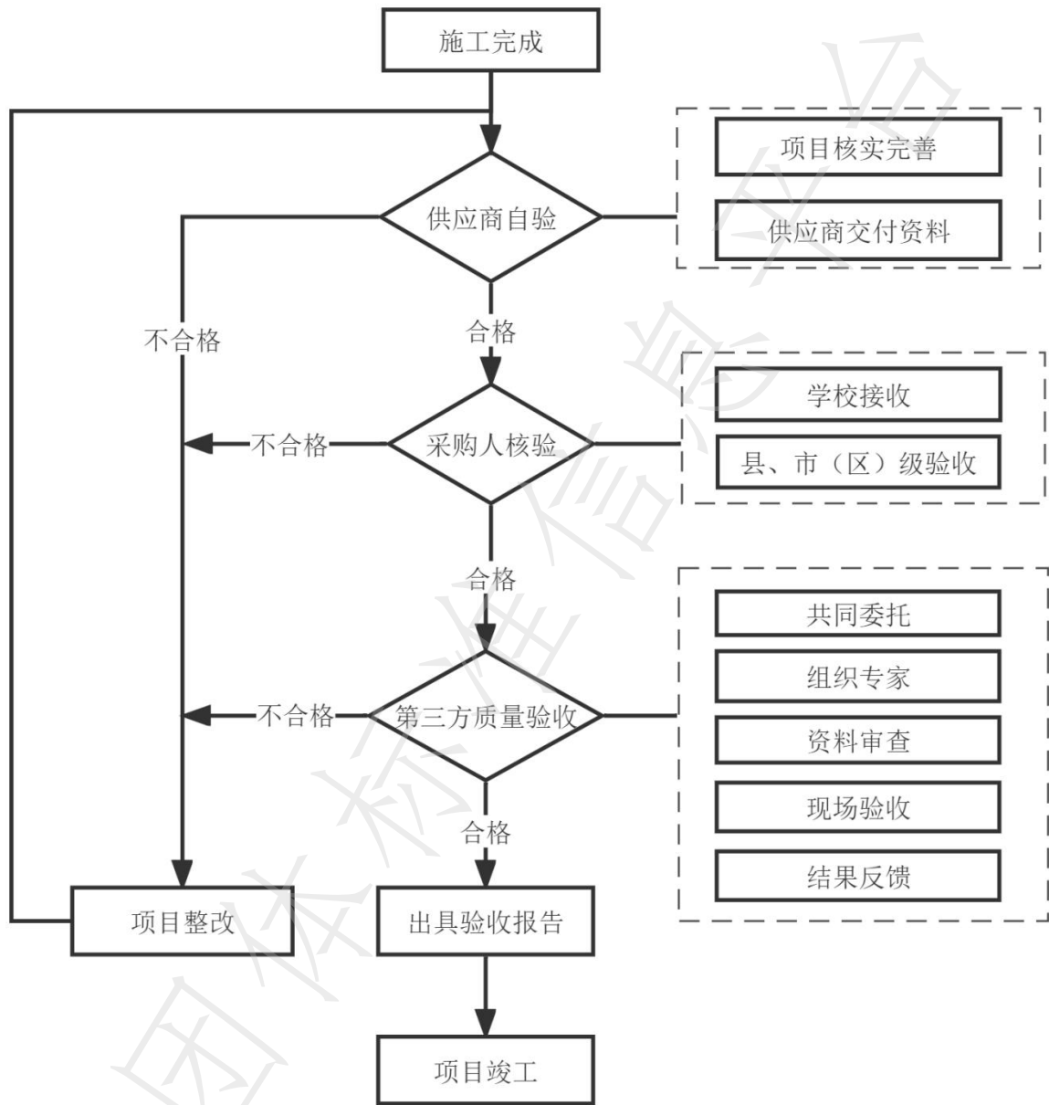
图 1 照明灯光验收流程示意图
