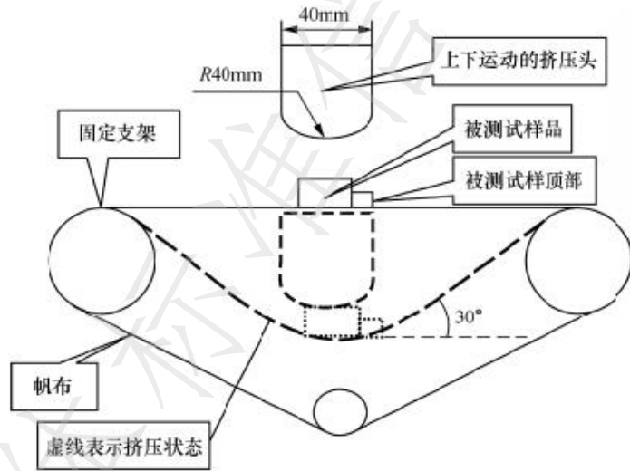
图2 试验示意图
