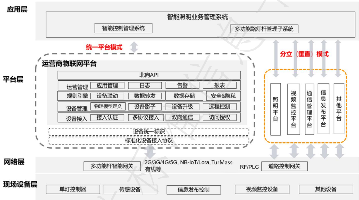
图A.1 智慧灯杆系统平台架构示意图
