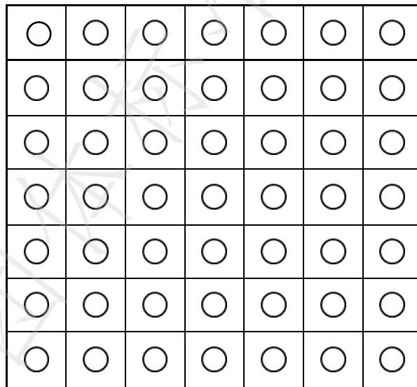
图B.1 教室一般照明照度测量网格中心布点示意图
