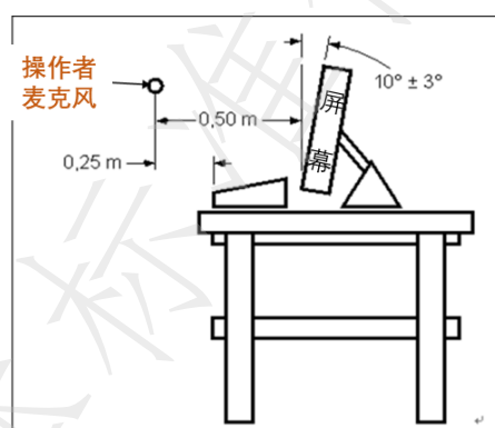
图 2 一体式微型计算机摆放示意图
