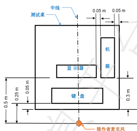
图 1- (b) 塔式系统摆放示意图
