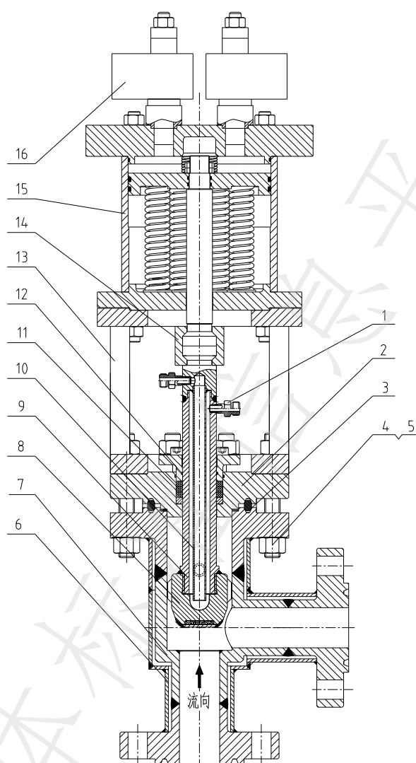
1. 冷却水接头 2. 阀盖 3. 八角垫 4. 螺柱 5. 螺母 6. 夹套 7. 阀体 8. 阀瓣 9. 阀杆 10. 芯管 11. 填料 12. O形橡胶圈 13. 支架 14. 哈弗连接套 15. 气缸 16. 快速排气阀
