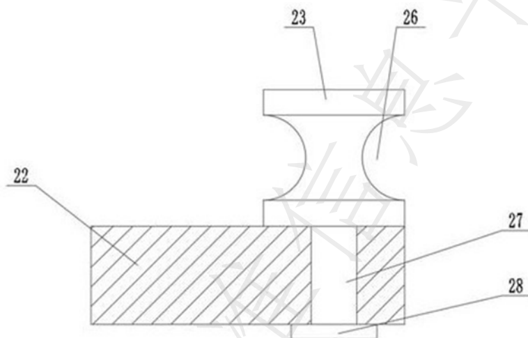
图2 软管承载机构示意图
