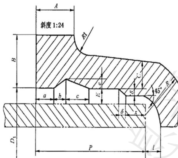
图5 承插式消防栓承插口连接尺寸
