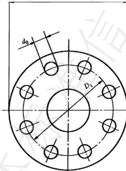
图4 法兰式消防栓法兰连接尺寸
