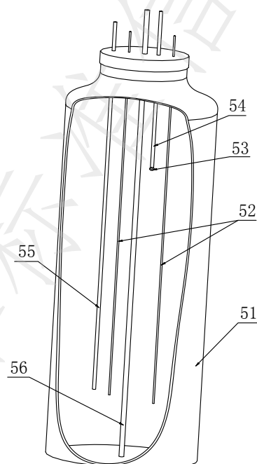
图 D. 7 热水管和常温水管的结构示意图
