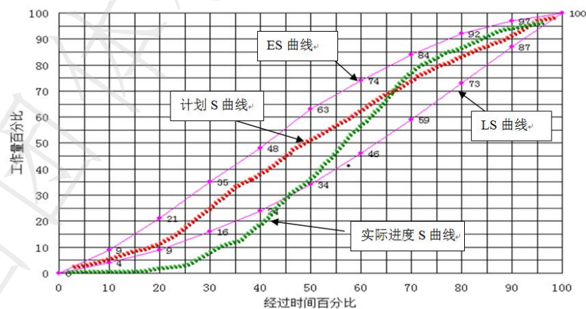
图4-1 进度管理曲线
