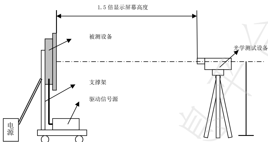
图 14 测量位置图
