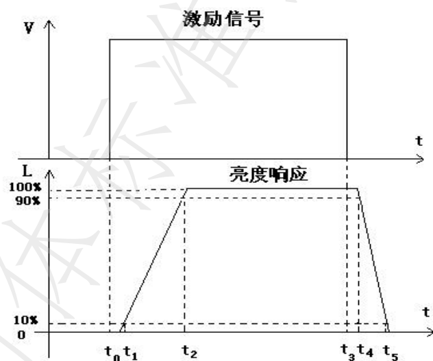
图 20 响应时间的测量
