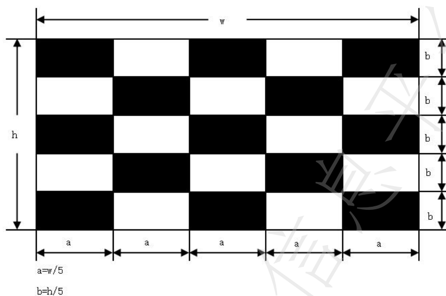
图 10 棋盘格信号
