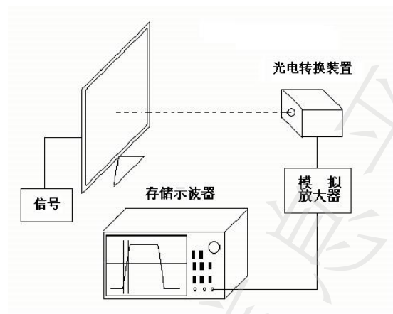
图 19 测试连接图
