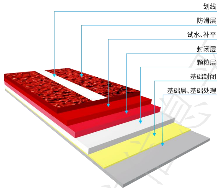
图6 复合型塑胶跑道分层结构图
