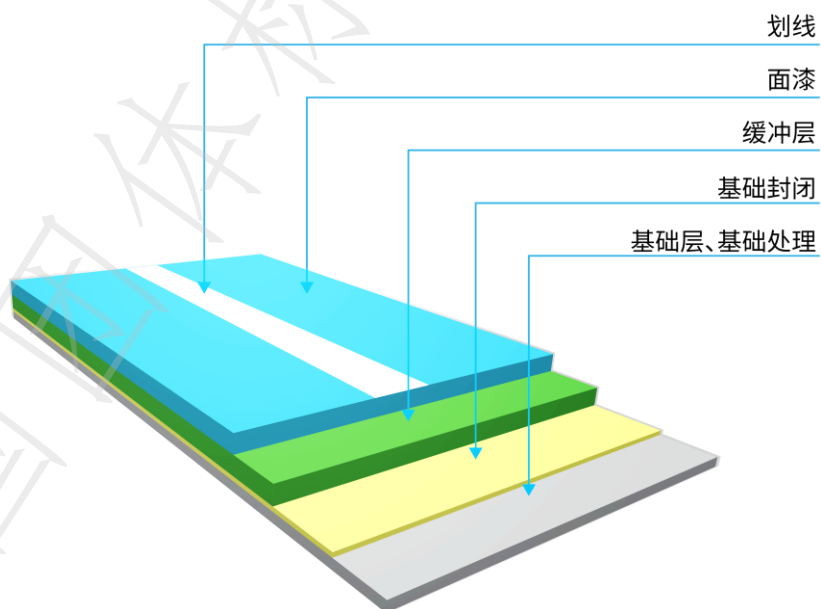
图10 聚氨酯球场分层结构图
