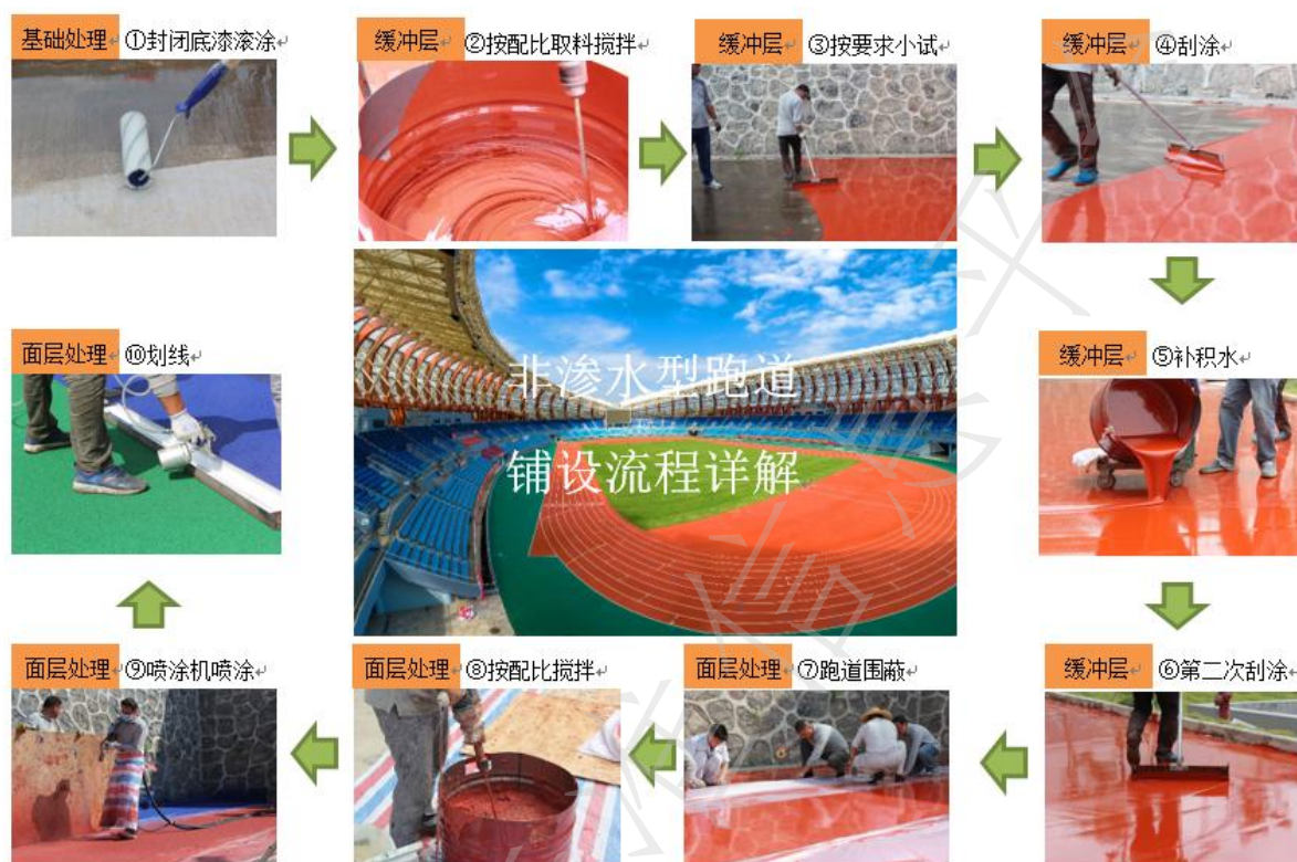
图7 非渗水型跑道铺设流程详解图
