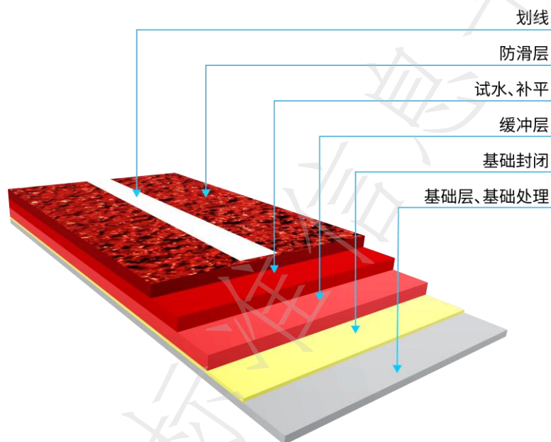
图4 全塑型塑胶跑道分层结构图
