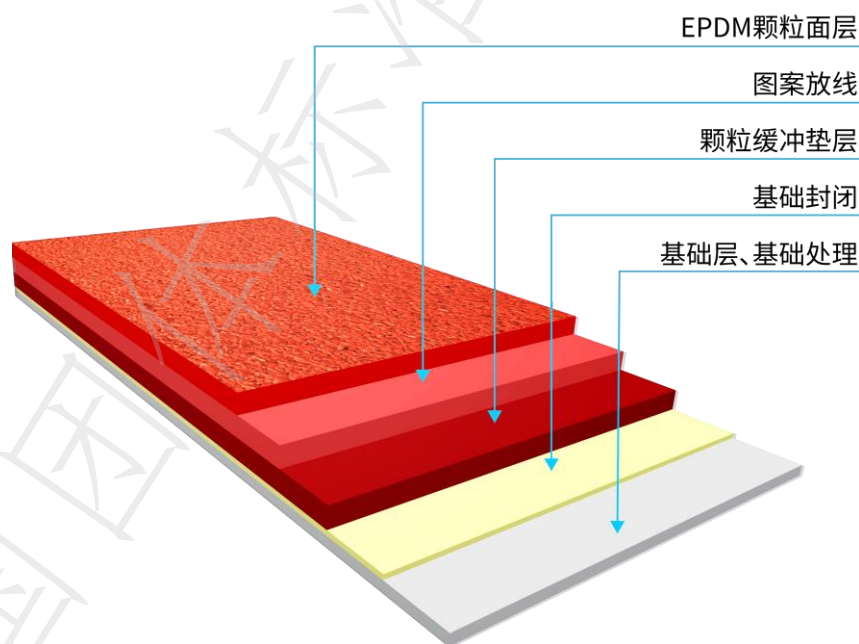
图13 彩色 EPDM 橡胶地垫分层结构图
