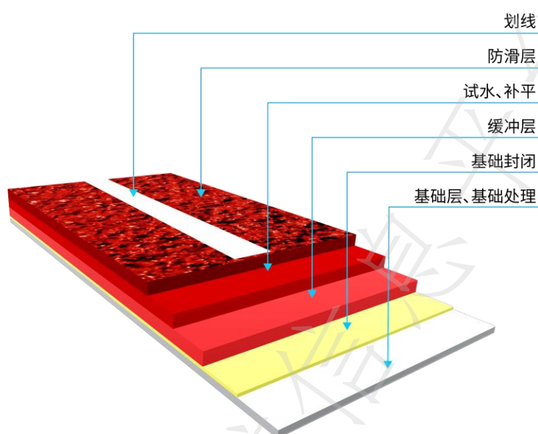
图5 混合型塑胶跑道分层结构图
