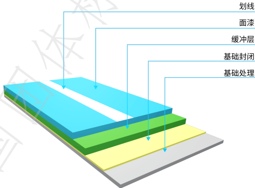
图12 硬地丙烯酸球场分层结构图
