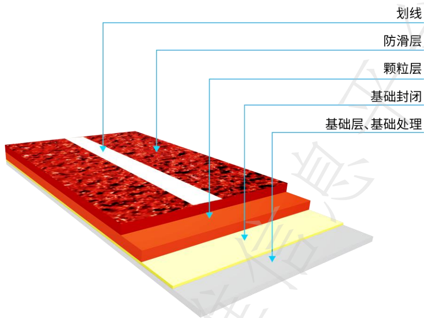
图8 透气型塑胶跑道分层结构图
