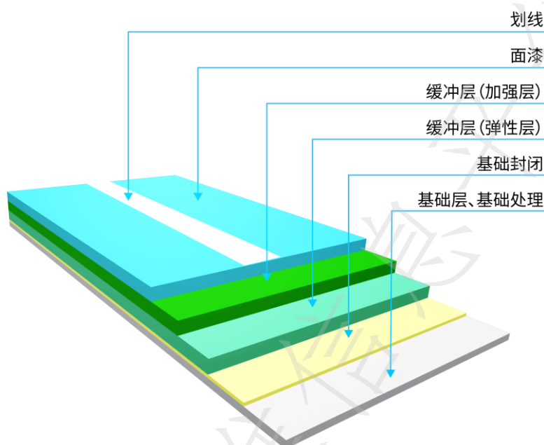
图11 弹性丙烯酸球场分层结构图
