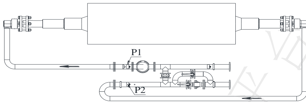
图3 陶瓷电晕辊的辊筒内水路通畅试验
