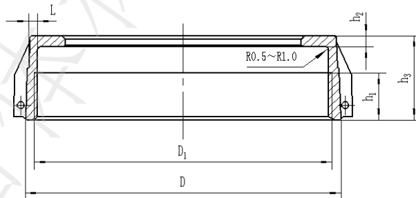
图A.3 湿式水表罩子
