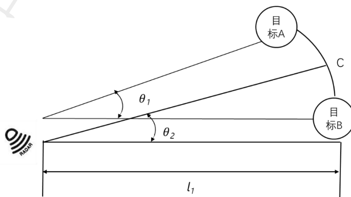
图 3 角度分辨力工况一
