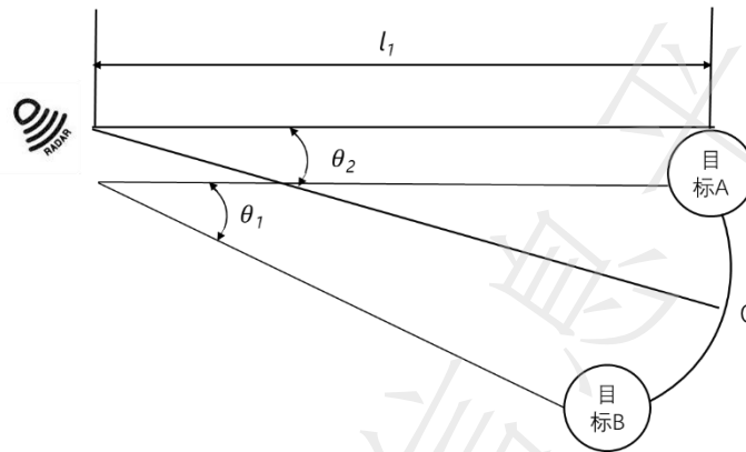
图 4 角度分辨力工况二
