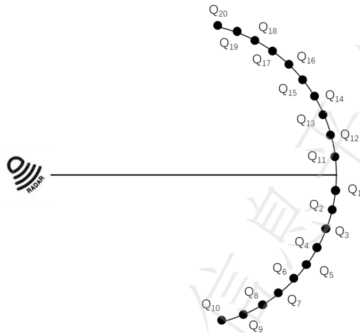
图 10 角度误差
