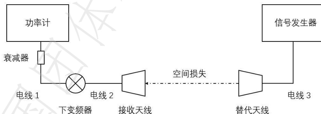
图 C.1 校准装置
