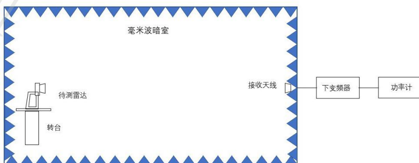
图 B.2 发射测试暗室
