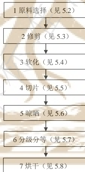
图1 “抚松人参”生晒参片加工程序流程图
