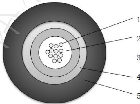
(1) 光纤; (2) 阻水填充物; (3) 松套管; (4) 玻璃纤维带(非金属纤维纱); (5) 护套。
