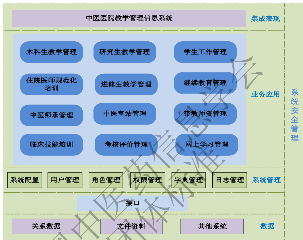
图A.1 中医医院教学管理信息系统功能架构
