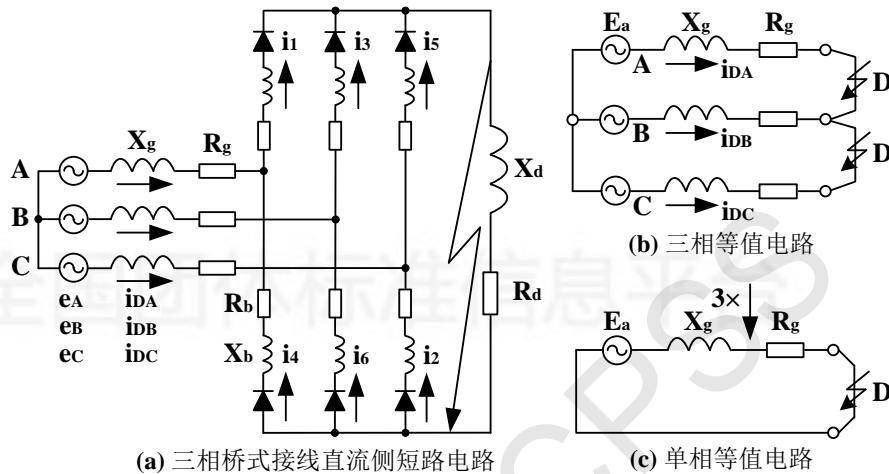
图 1 三相桥式接线直流侧短路电路
