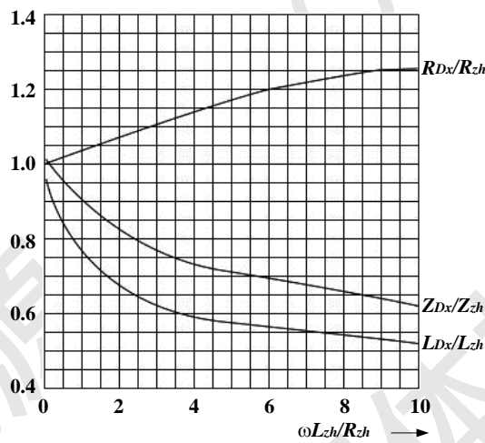
图4 等效阻抗 Z_{Dx} 系数曲线
