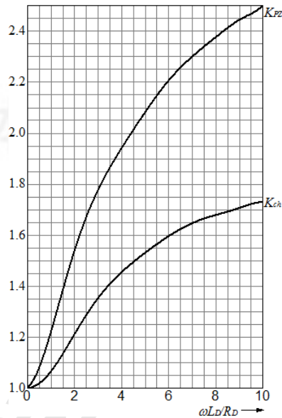
图 2 冲击值暂态系数曲线
