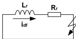
图 8 高压开关断开后的等效电路模型
