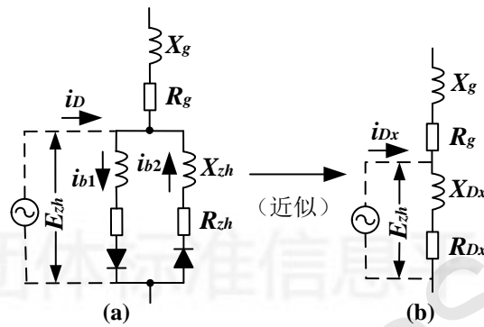
图3 确定等效分支阻抗 Z_{Dx} 的的等值电路
