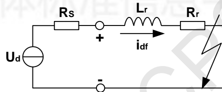
图 7 三相桥式变流器经直流电抗器后短路的等效电路模型
