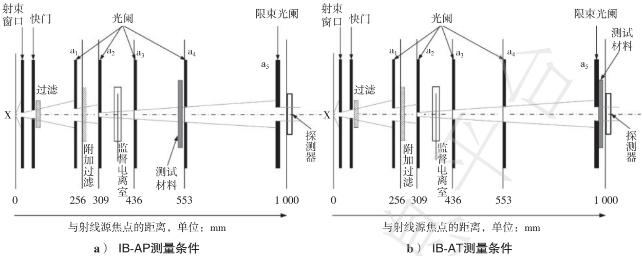
图4 改进的逆宽射束测量条件示意图
