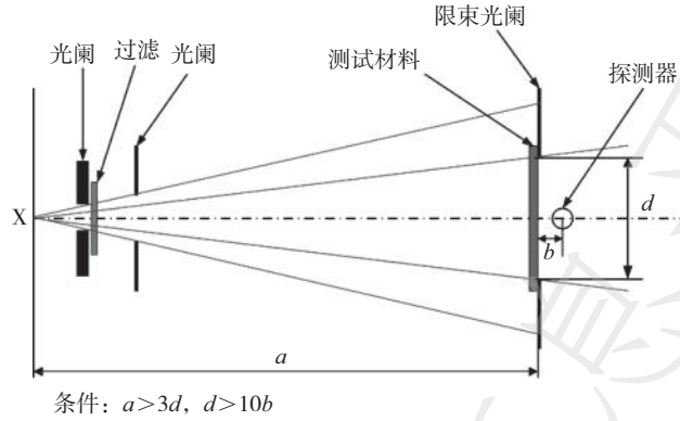
图2 宽射束测量条件示意图
