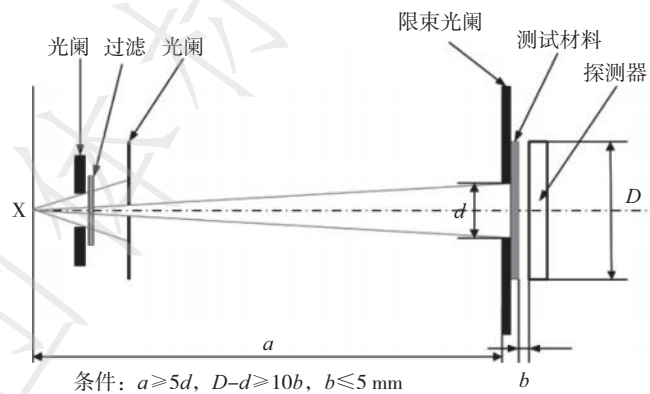
图3 逆宽射束测量条件示意图
