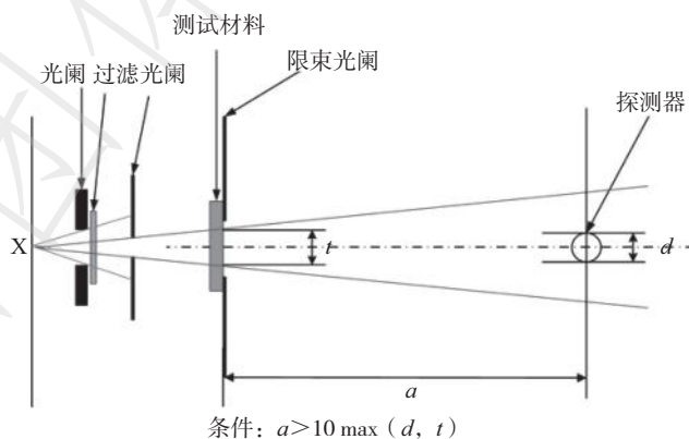
图 1 窄射束测量条件示意图
