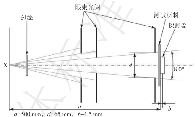
图5 改进的宽射束条件示意图
