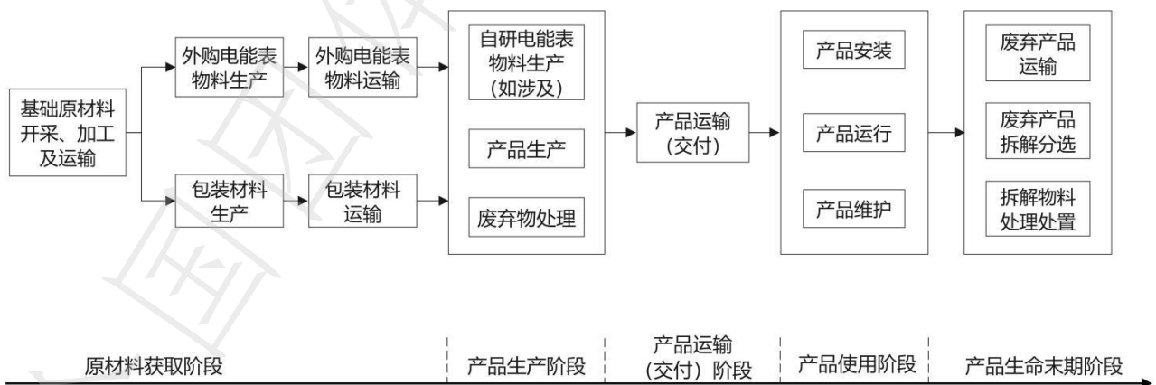
图 1 电能表产品碳足迹系统边界示意图
