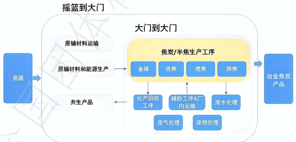
图 1 冶金焦炭产品系统边界图
