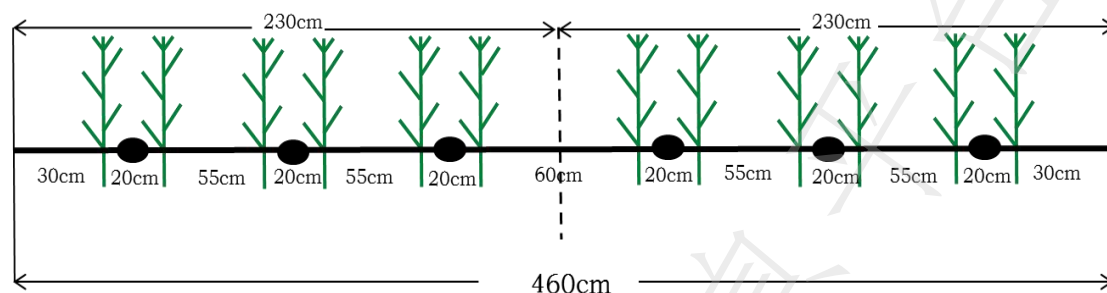
图 1 田间种植方式示意图（一机两膜）
