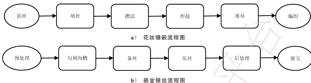
图1 金银丝镶嵌工艺流程示意图
