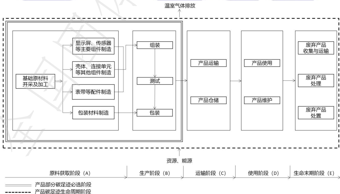
图 1 智能手表产品碳足迹量化系统边界
