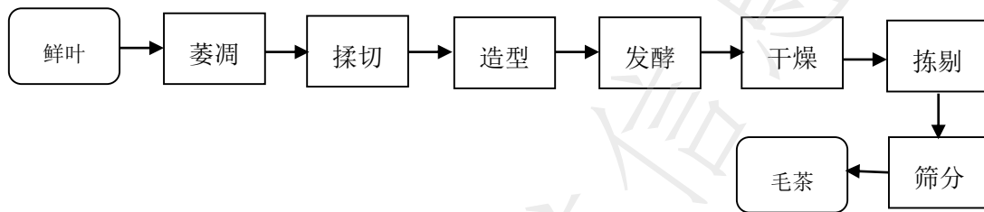
图1 红碎茶加工工艺流程图
