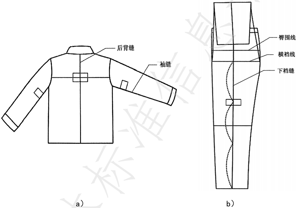
图 D.1 接缝处纱线滑移取样示意图
