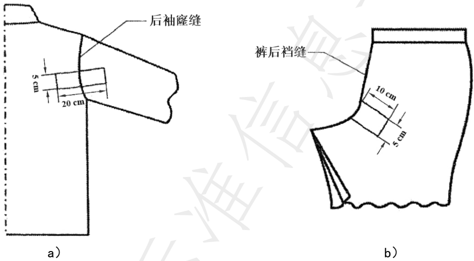
图 E.1 接缝强力取样示意图
