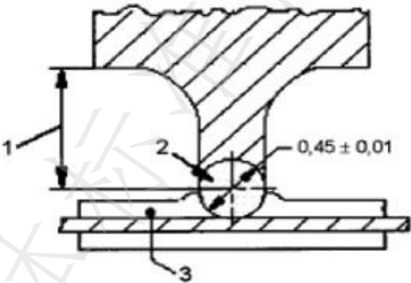
图 E.1 动态穿透试验装置
