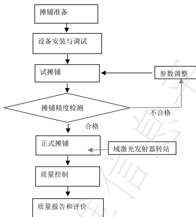
图1 工艺流程
