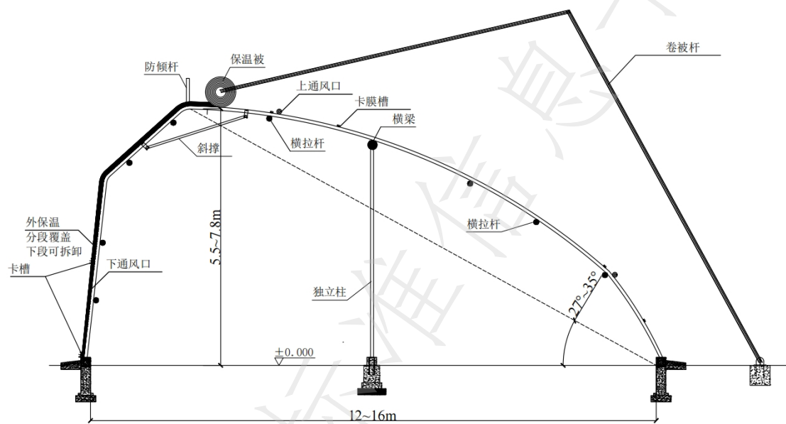
图 A 大跨度保温型日光温室剖面示意图
