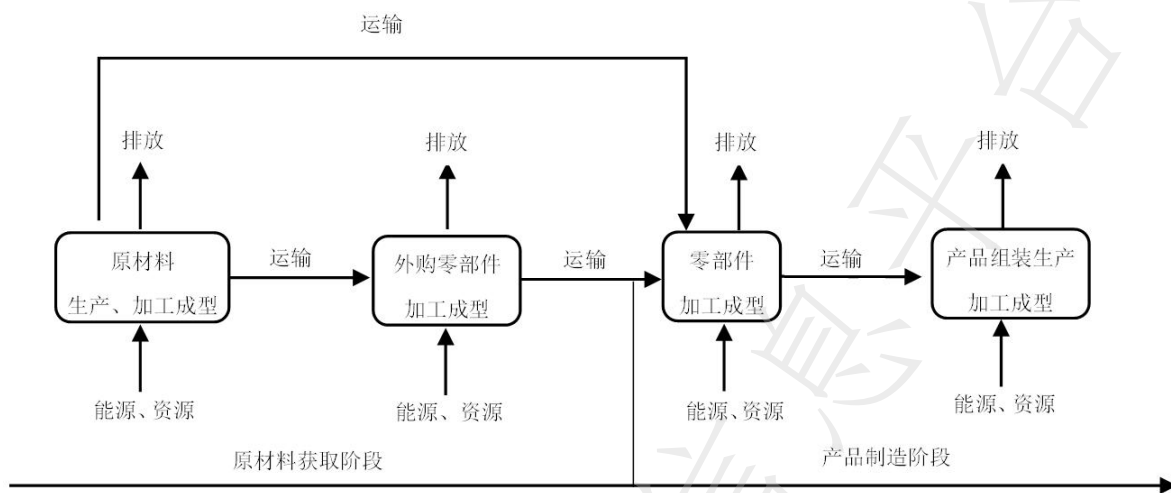
图1 小功率电动机产品碳足迹量化的系统边界示例
