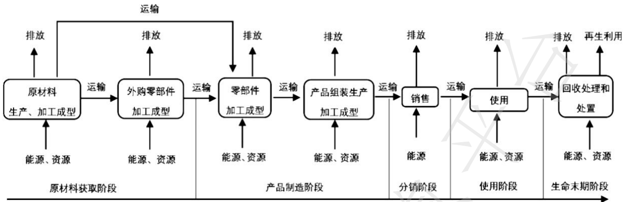
图1 吸油烟机产品碳足迹量化的系统边界示例
