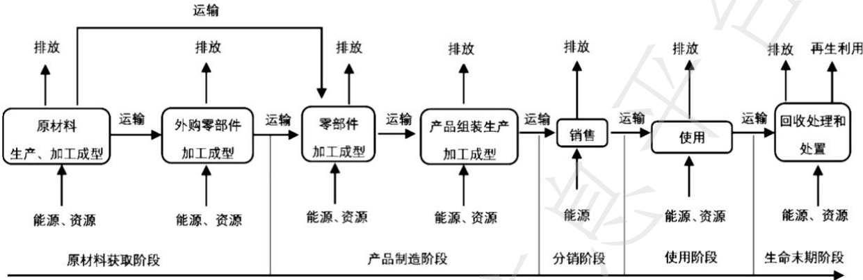
图1 储水式电热水器产品碳足迹量化的系统边界示例
