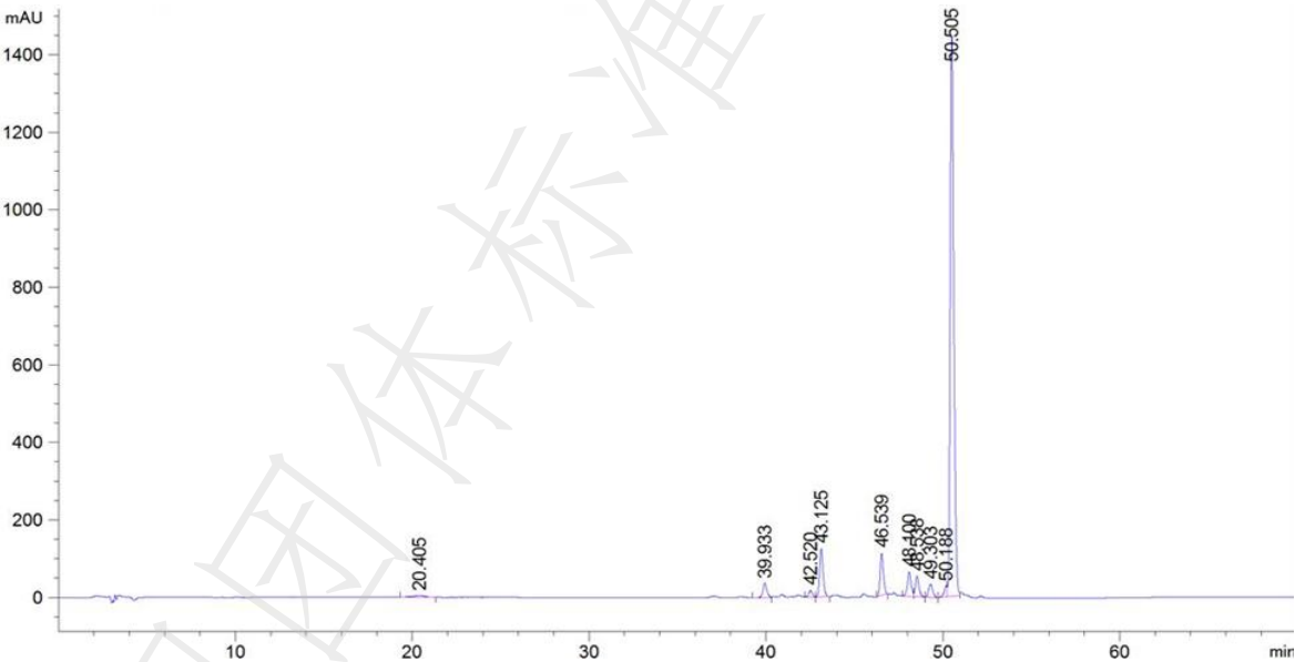
图 A.1 玉米黄素双棕榈酸酯标准物质的 HPLC 图谱
