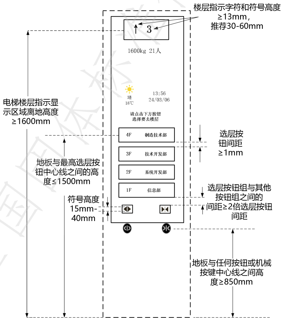
图4 轿内触摸屏示意
