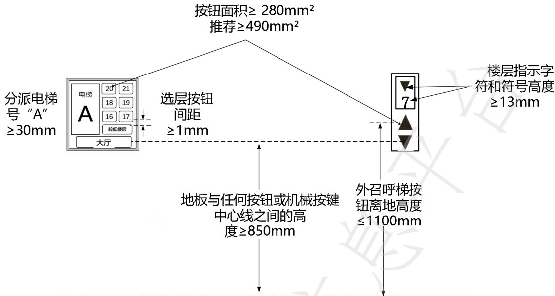
图3 层站触摸屏示意（左：乘梯分派，右：外招呼梯）
