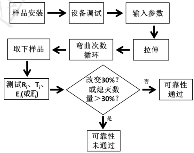
图4 试验流程图
