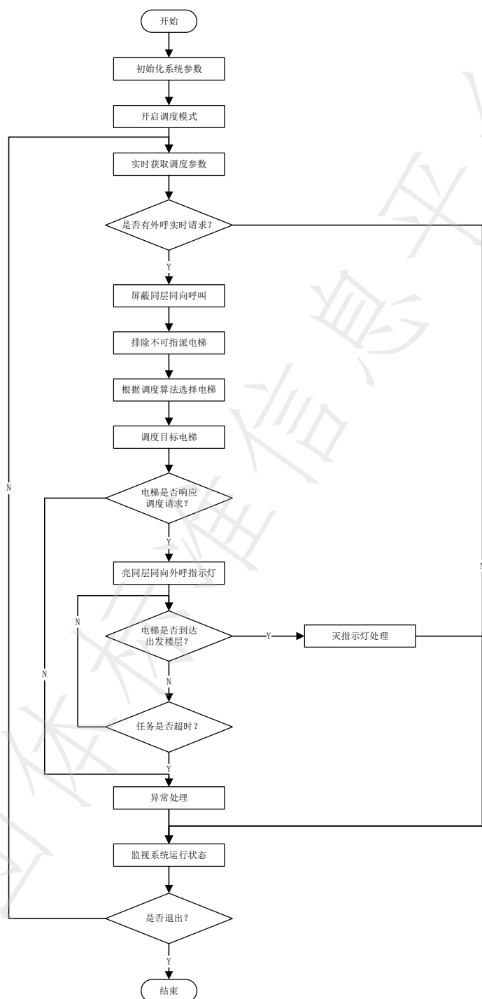
图4 调度流程图
